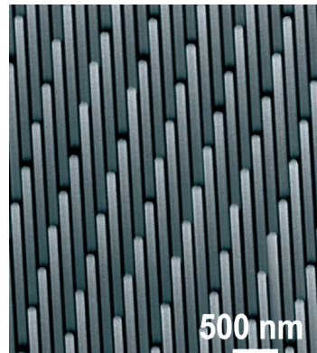
半導体ナノワイヤアレイ
