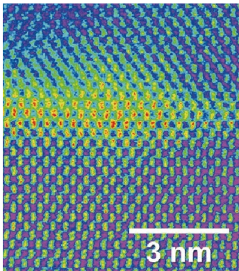
作製したナノ材料の電子顕微鏡写真
