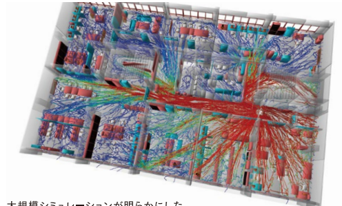
大規模シミュレーションが明らかにした 無線LANアクセスポイントから放射する電波の伝搬路
