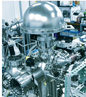
マグネタイト表面の計測システム
