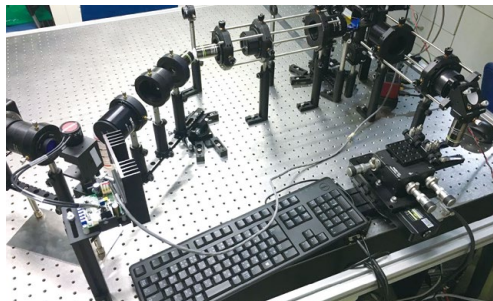
超高速3D蛍光顕微鏡
