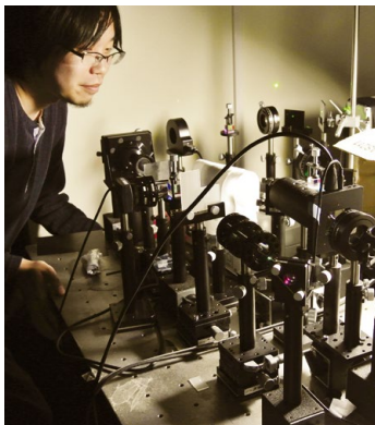
位相共役光による生体イメージング
